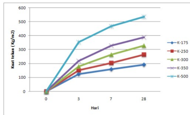
Grafik Kuat Tekan BEPMIX
